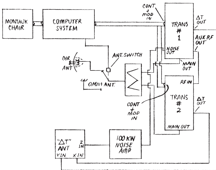
ОБЩА БЛОК-СХЕМА
